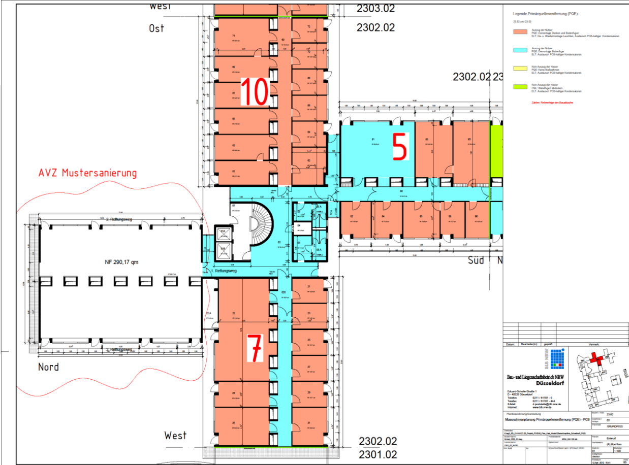
Gebäudeteil 23.02.02
